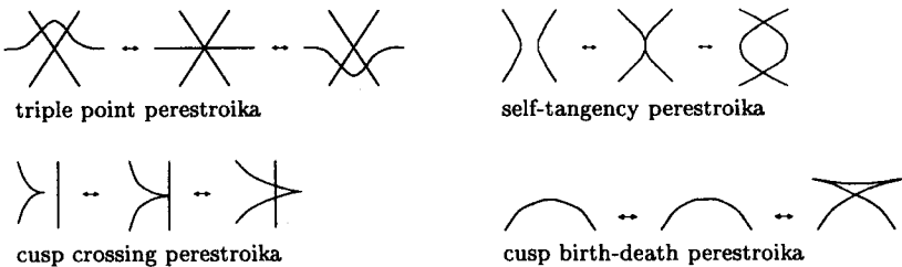
Fig. 3. Perestroikas
