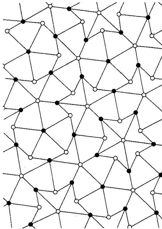
Figur 15: Penrose-Parkettierung mit “Kites” und “Darts”
